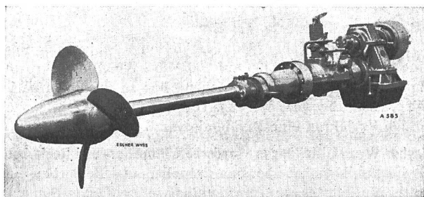
Abb. 2 Verstellbarer Schiffspropeller
