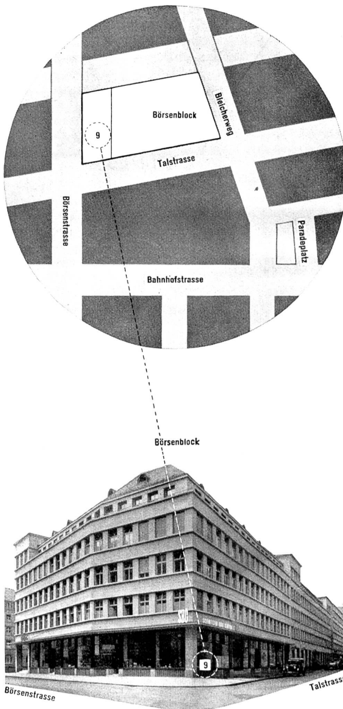
Fig. 21 Situationsplan und Aussenansicht der Schweizer Baumuster-Centrale. Plan de Situation et vue extérieure de l'Exposition permanente des matériaux de construction.
