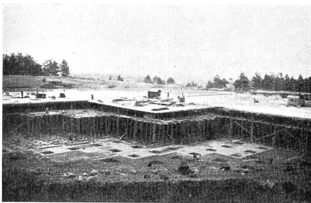
Abb. 3 Reservoir der Wiener Wasserversorgung im Lainzer Tiergarten (Nutzinhalt 144.000 m 3 ).
