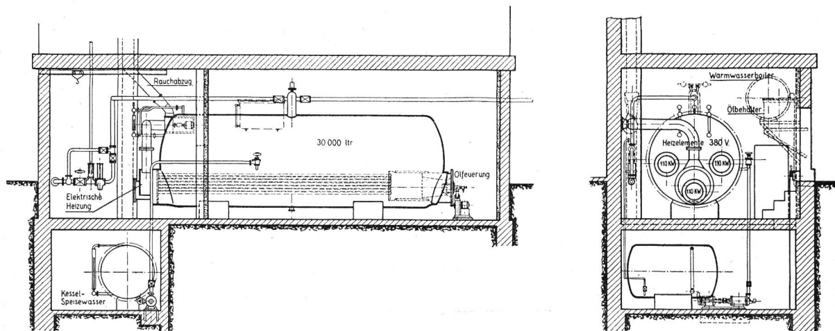
Abb. 13 Schlachthaus der Stadt Aarau. Längs- und Querschnitt durch den Elektro-Oeldampfkessel. Maßstab 1 : 300
