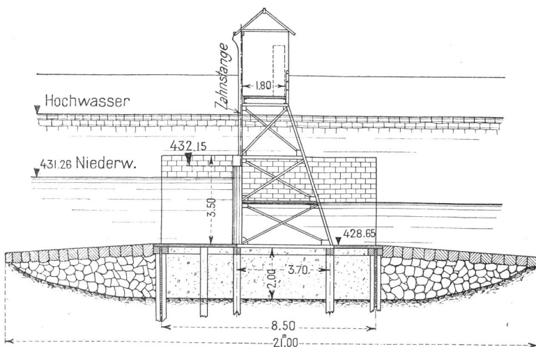
Abb. 3. Die Vergrößerung des Niederwasserabflusses aus den Juraseen. Das Nidauerwehr vor dem Umbau. Querschnitt durch die Seitenöffnung. 1:200.
