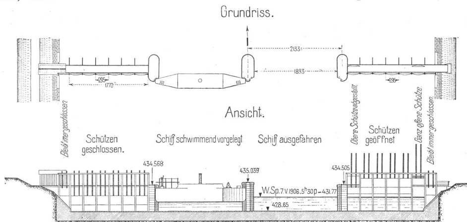
Abb. 1. Die Vergrößerung des Niederwasserabflusses aus den Juraseen. Das Nidauerwehr vor dem Umbau. Ansicht und Grundriss. 1:800.
