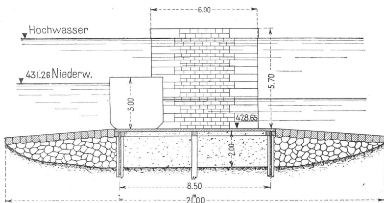
Abb. 2. Die Vergrößerung des Niederwasserabflusses aus den Juraseen. Das Nidauerwehr vor dem Umbau. Querschnitt durch die Mittelloffnung. 1:200.
