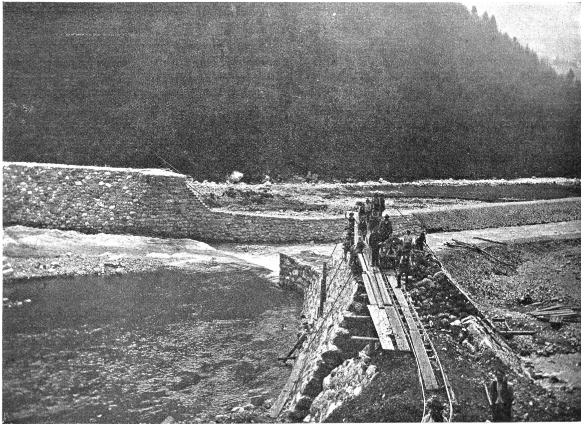
Die Muotakorrekction. Abb. 5. Erstellung des rechtseitigen Abschlussdammes in der „Balm“
