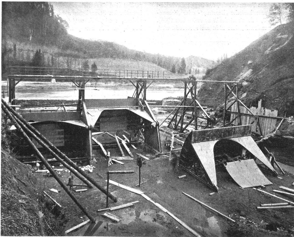
Abbildung 2. Segmentschützwehr bei Hauterive (Freiburg).
