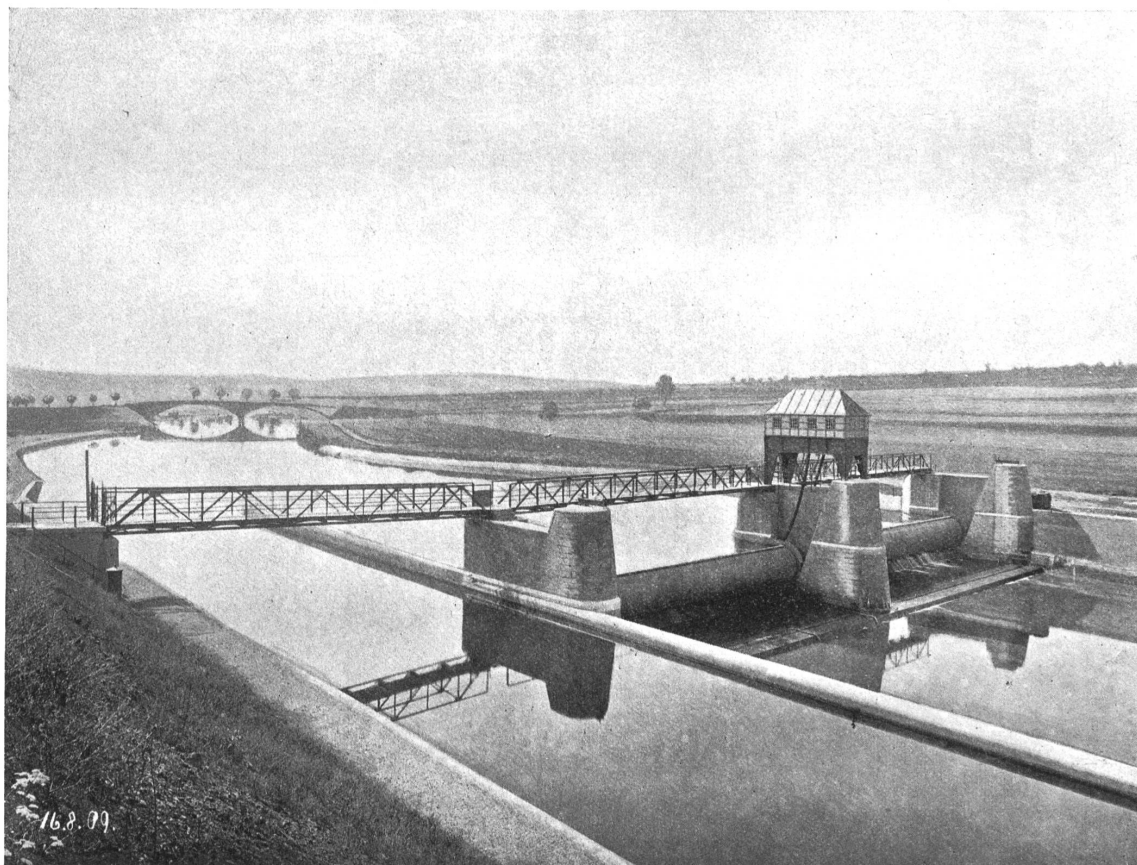
Abbildung 1. Walzenwehr Pöppelweiler (Württemberg).
