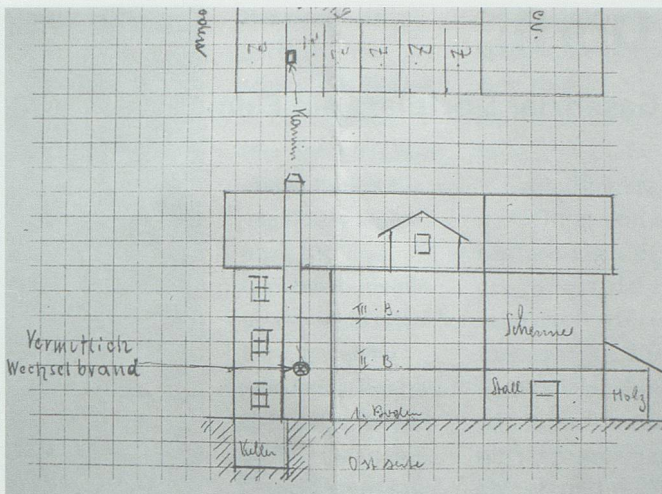
«Vermutlich Wechselbrand» in der Balkenlage zum 1. Stock des Gebäudes: Zeichnung von Baumeister und Feuerwehrkommandant Matthias Gabathuler, Oberschan, in dessen Brandrapport.
