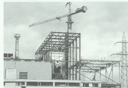
9. Juni: Die Ofenlinien 1 und 2 der Kehrrechtverbrennungsanlage Buchs werden für rund 13,1 Millionen Franken nachgerüstet.
