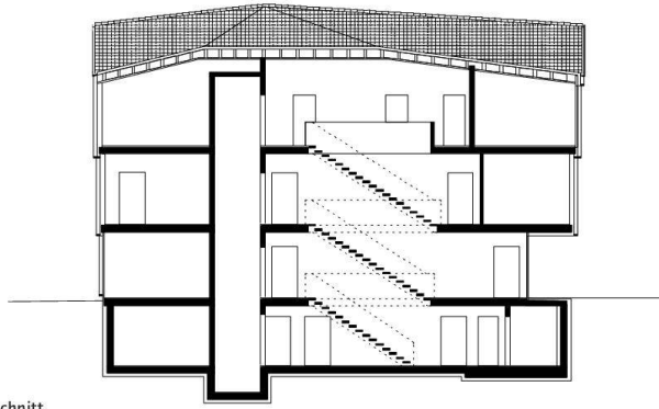
Längsschnitt
