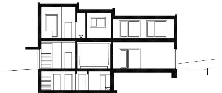
Schnitt A-A
