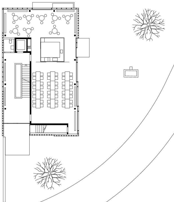
Erdgeschoss
