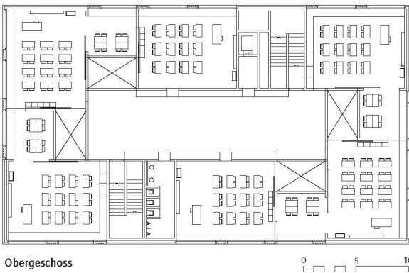
Obergeschoss
