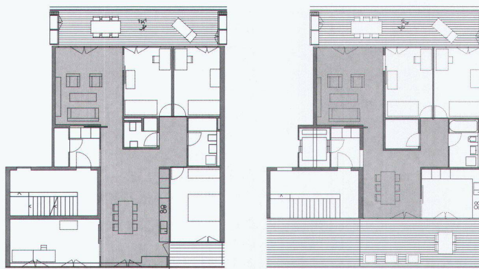
5 1/2- und 3 1/2-Zimmerwohnung
