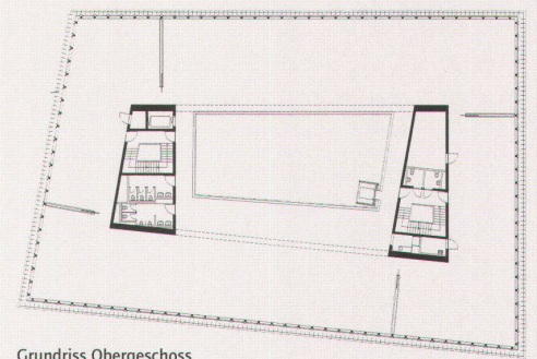
Grundriss Obergeschoss
