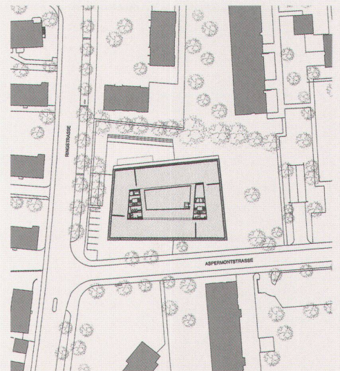
Lageplan
