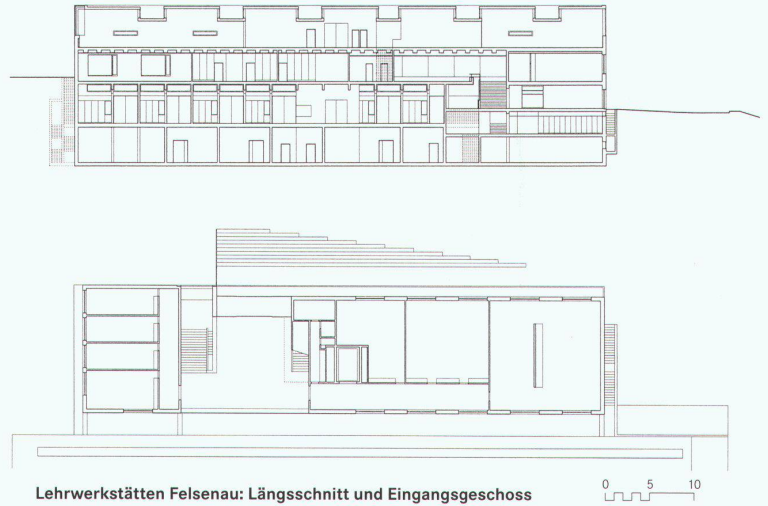
Lehrwerkstätten Felsenau: Längsschnitt und Eingangsgeschoss
