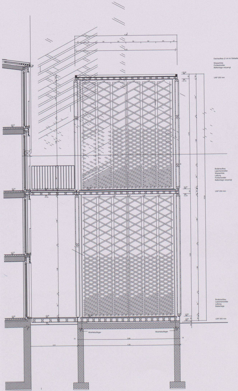
Schnitt Laubenturm
