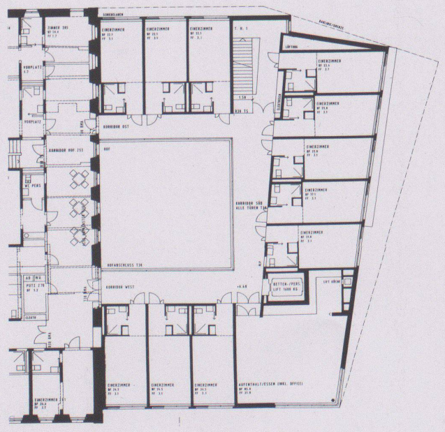
1. und 2. Obergeschoss
