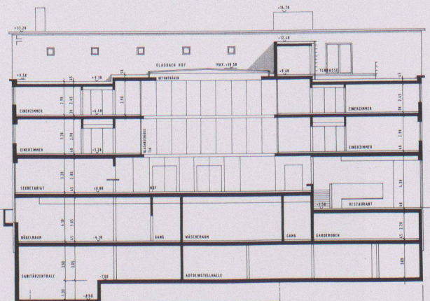
Schnitt Ost/West
