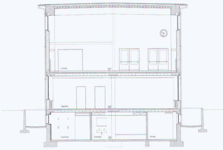
Schnitt durch den Saaltrakt. Projektplan, 2001 0 100 200
