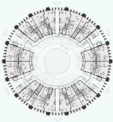
Regelgrundriss
