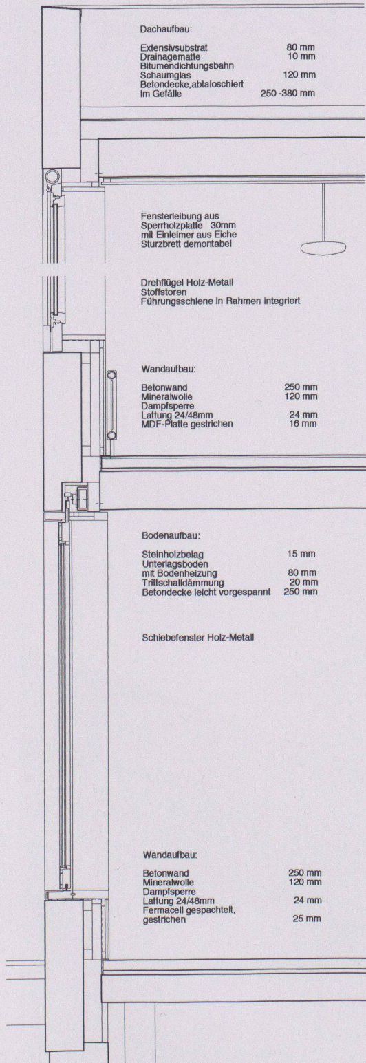
Schnitt Aussenfassade
