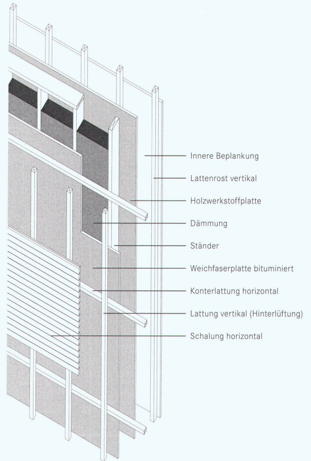
Holzrahmenbau, Axonometrie
