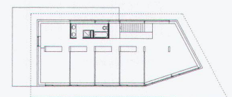
Obergeschoss
