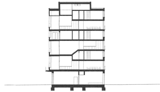
Querschnitt
