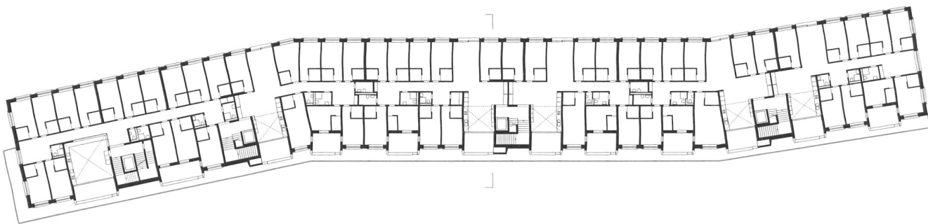
1. Obergeschoss
