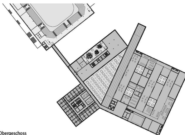
Obergeschoss
