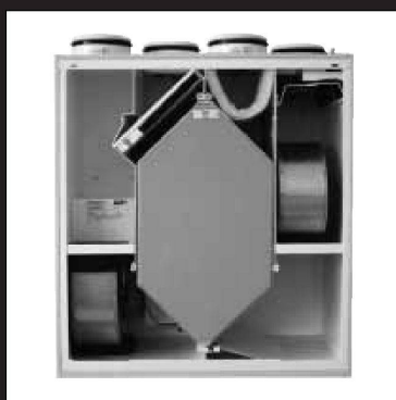
KWL-Lüftungssystem
