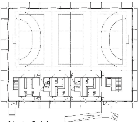
Erdgeschoss Turnhalle
