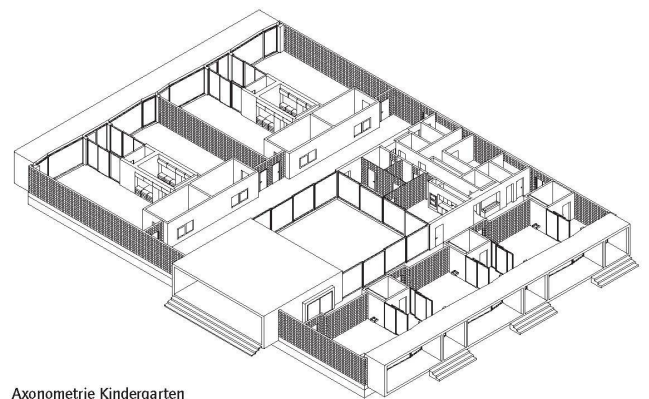
Axometrie Kindergarten
