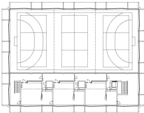
Obergeschoss Turnhalle
