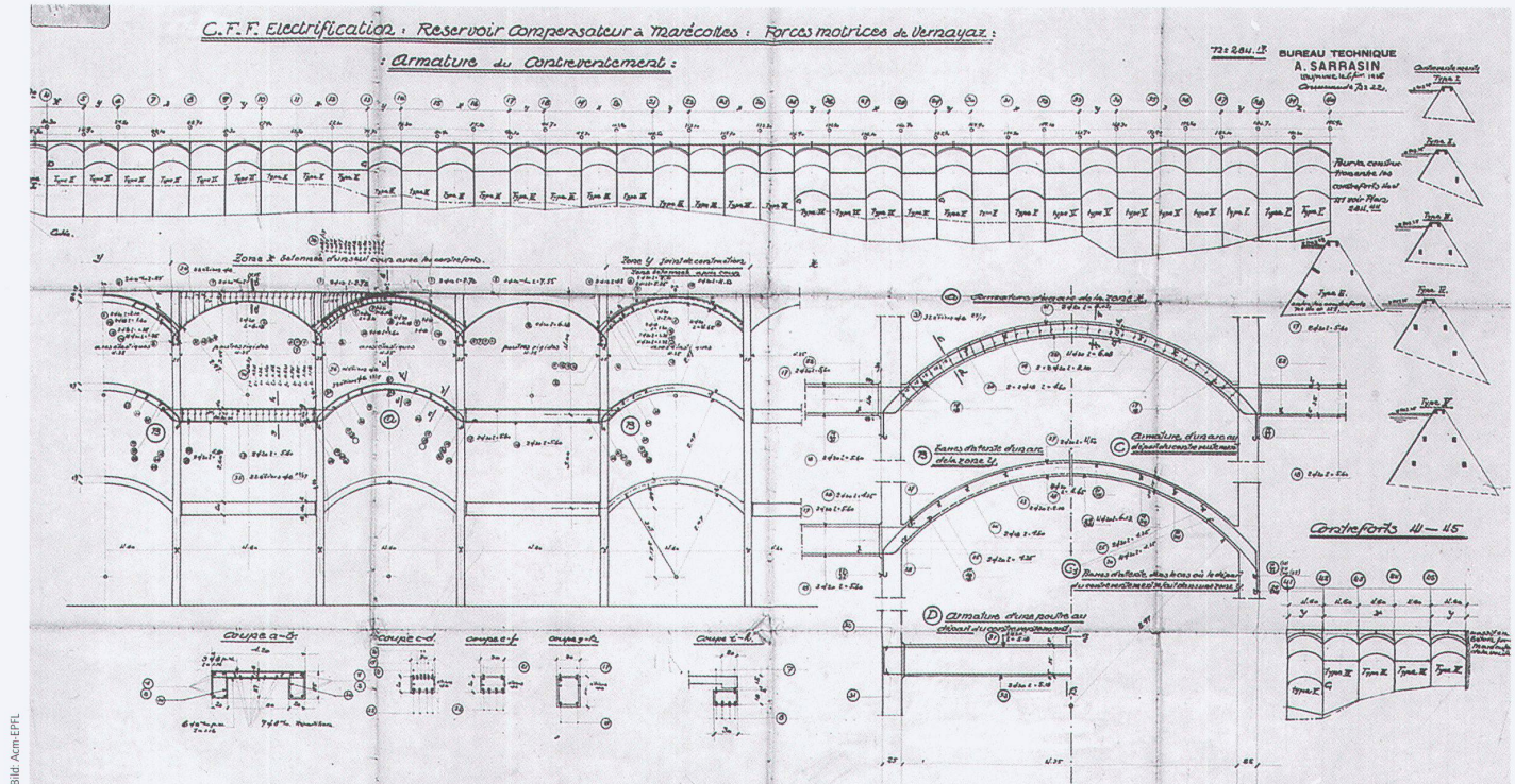
Ausgleichsbecken Les Marécottes (VS), 1925, Ing. Alexandre Sarrazin. Acm-EPFL, fonds Sarrazin.
