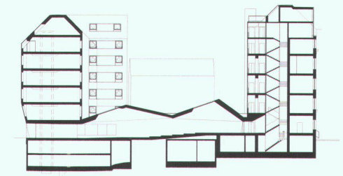
Längsschnitt durch Vortragssaal
