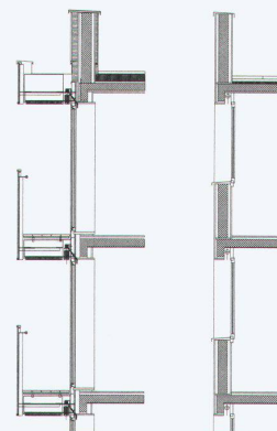
Fassadenschnitt neu
