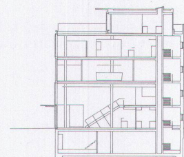
Längsschnitt
