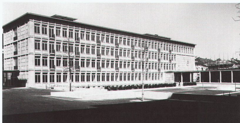
Basel, Architekturmuseum: Real-Gymnasium 1954/57, Klassentrakt mit Pausenhof; Architekten: Ernst Mumenthaler und Otto Meier
