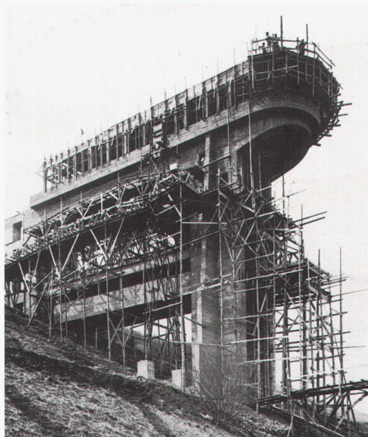
Zürich, ETH Zentrum: Maurice Braillard, Drahtseilbahn von Salève 1931–1932, Bergstation im Bau
