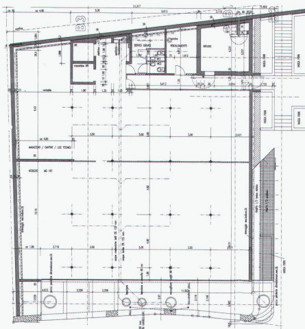
Sockelgeschoss (Parkgarage) und Aufsicht ■ Soubassement (garage-parking) et vue de dessus ■ Base floor (parking garage) and plan view
