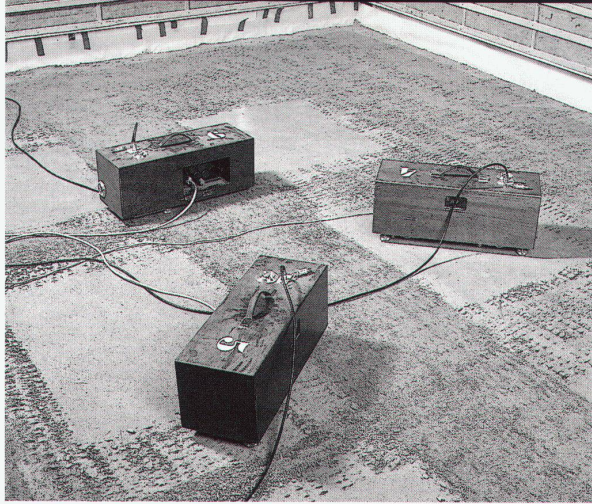
Trittschallprüfung mit Klopfggeräten unter realen Baubedingungen (Unterlagsboden vollflächig, lange Belastungsdauer) in der EMPA Zürich.
