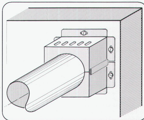
Rohrmanschetten PROMASTOP, S90 für D = 50 - 200 mm
