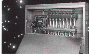
Die kompakte Lösung: Verteilerkasten Tacobioc, Beulco-Verteiler.
