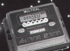
Präzis und unbestechlich: Wärmezähler Multical mit Dialog- system.
