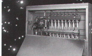
Die kompakte Lösung: Verteilerkasten Tacobloc, Beulco-Verteiler.
