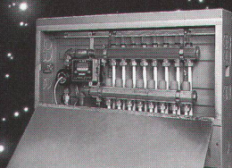
Die kompakte Lösung: Verteilerkasten Tacobloc, Beulco-Verteiler.
