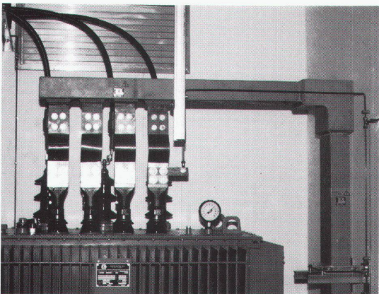
Trafoanschluss mit Betobarschiene 1000 A
