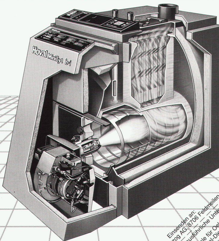
Kompakt-Wärmezentrale Hoval MiniLyt b-i.
