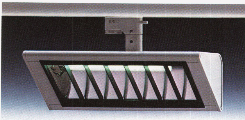
Optec-Wandfluter für kompakte Leuchtstofflampen sind 330 mm breit. Für gleichmäßige Beleuchtungsstärken zwischen 50 und 100 Lux werden sie mit 7 W-, 9 W- und 11 W-Lampen ausgerüstet. Blendschutzraster gewährleisten hohen Sehkomfort und UV-Filterfolien höchsten Lichtschutz.
