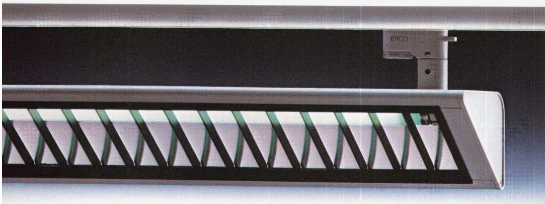
Optec-Wandfluter für 26 mm Leuchtstofflampen der Leistung 18 W sind 700 mm breit. Sie werden für gleichmäßige Wandbeleuchtungen bis 150 Lux eingesetzt. Auch hierfür bieten Blendschutzraster hohen Sehkomfort und UV-Filterfolien ausreichenden Lichtschutz.
