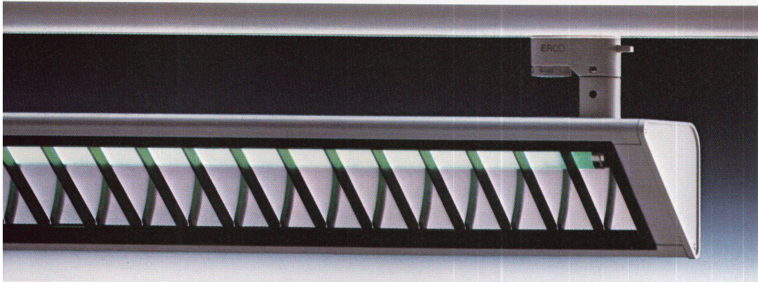
Optec-Wandfluter für 26 mm Leuchtstofflampen der Leistung 36 W sind 1300 mm breit. Damit lassen sich gleichmäßige Beleuchtungsstärken von 300 Lux erreichen. Auch hierbei gehören Blendschutzraster und UV-Lichtschutzfilter zum Lieferumfang.
