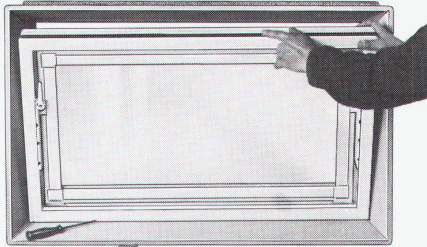
Inset Kellerfenster Plast/Kipp
