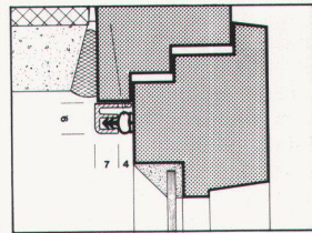
Fenstersanierung HEBCO 121/526
