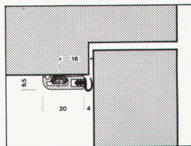
Türsanierung HEBCO 126/631
