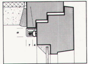
Fenstersanierung HEBGO 121/526
