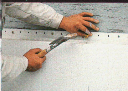
Setzen des Schlagdübels.
