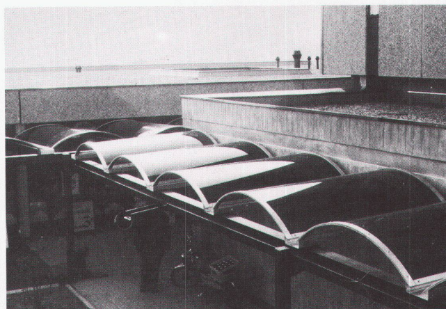
Teilansicht des 220 m 2 Vordaches aus getöntem Polycarbonat Einkaufszentrum Marly-Fribourg
