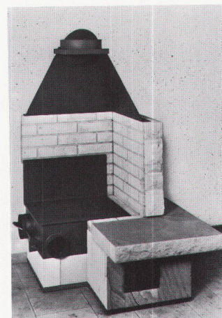
Frei-Mini-Warmlufteinsatz für den nachträglichen Einbau mit eingebautem Ventilator
