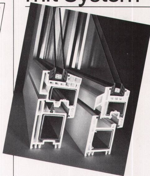
2flügliges Dreh-/Kippfenster ohne Setztück
