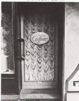
...ohne Stolperschwellen...
