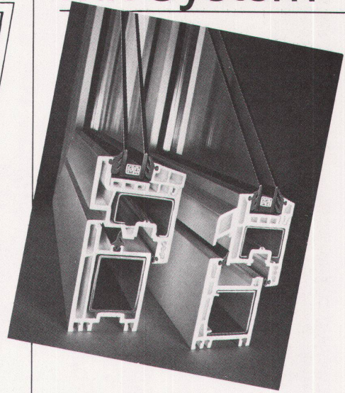
2flügeliges Dreh-/Kippfenster ohne Setztstück
