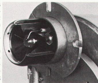
Schnittbild eines Kleinstflammpfropfes mit deutlich sichtbarer Minidüse. Im aufgeschnittenen Flammrohr erkennbar die Austrittsöffnungen für die vorgewärmte Verbrennungsluft. Sie erlaubt eine vollständige Verbrennung und hohe Wirtschaftlichkeit.
