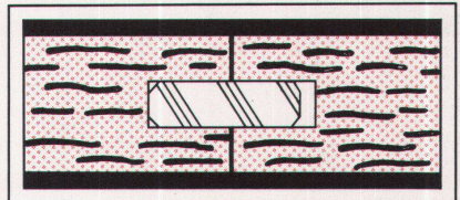
Die geruchsfreien NOVOPAN-Wand- und Bodenplatten sind ringsum genestet. Für 4-mm-Federn.
