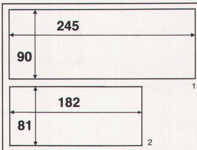
1 Wandplatte 2 Bodenplatte
