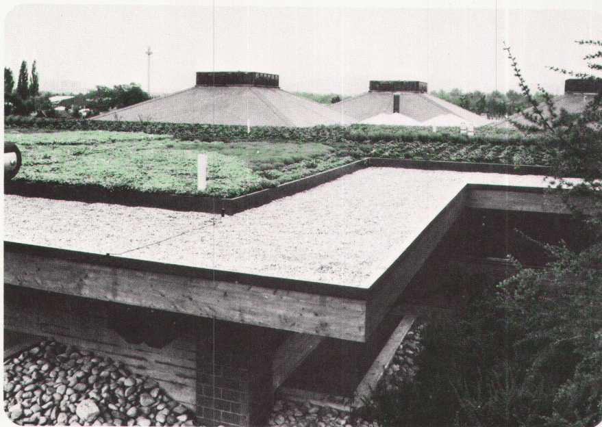
Objekt: Restaurant Seegarten, Park im Grünen, Grün 80, ca. 750m 2 Dachbegrünung, Schichthöhe 17cm. Planung: Architekten Rasser und Vadi, Basel und S.u.M. Zürich. Gartenarchitekten W. Neukom, Zürich und A. Zürcher, Oberwil ZG. Ausführung: Bieber Gartenbau AG , Rheinfelden.
